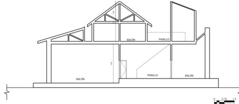
Corte longitudinal
